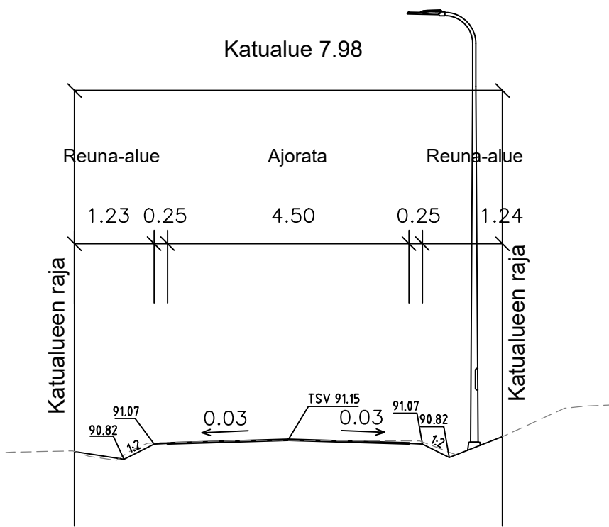
TYYPPIPOIKKILEIKKAUS 1:100 Peltokummuntie (pl 90)
