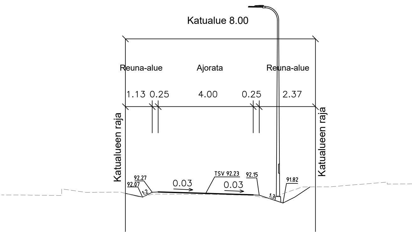
TYYPPIPOIKKILEIKKAUS 1:100 Kumpukuja (pl 40)
