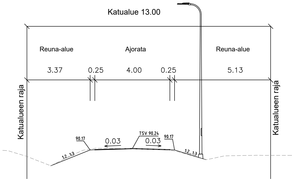
TYYPPIPOIKKILEIKKAUS 1:100 Läntinenkatu (pl 80)
