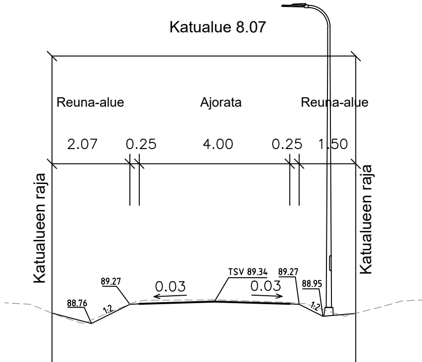
TYYPPIPOIKKILEIKKAUS 1:100 Läntinenkatu (pl 140)
