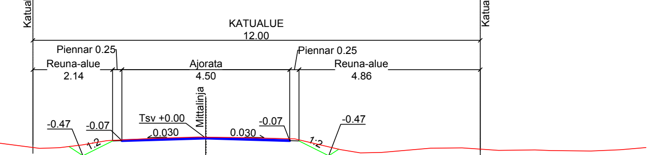
PELTOKUMMUNTIE TYYPIPOIKKILEIKKAUS 1:100 PL 100
