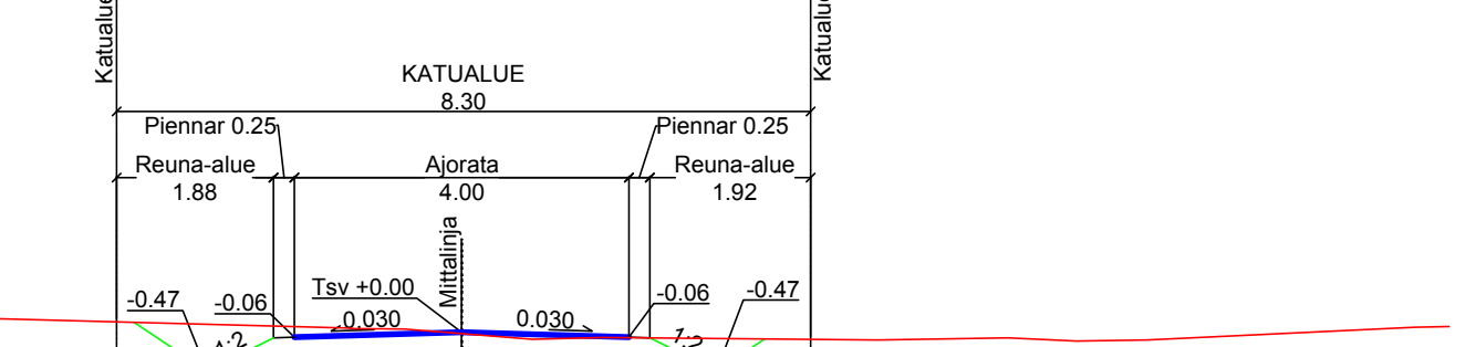
METSÄTIE TYYPIPOIKKILEIKKAUS 1:100 PL 510
