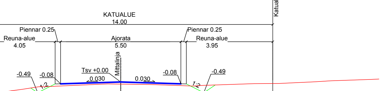
METSÄLÄNTIE TYYPIPOIKKILEIKKAUS 1:100 PL 390
